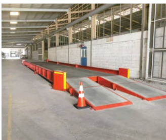
ပြောင်းလဲသည့်ချိန်ကိရိယာ CTS မော်ဒယ်
