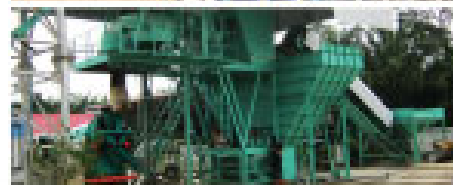
แบบปั๊ม รุ่น Packet Silo Type (ใช้รถเท 10 ตัน)
