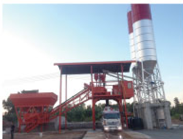
แบบปั๊ม รุ่น Semi Mobile Type - I (พร้อม ไมโคร 1)
