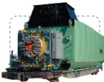
ໝໍ້ໄອນ້ຳແບບທໍ່ນ້ຳຄວາມດັນສູງ
